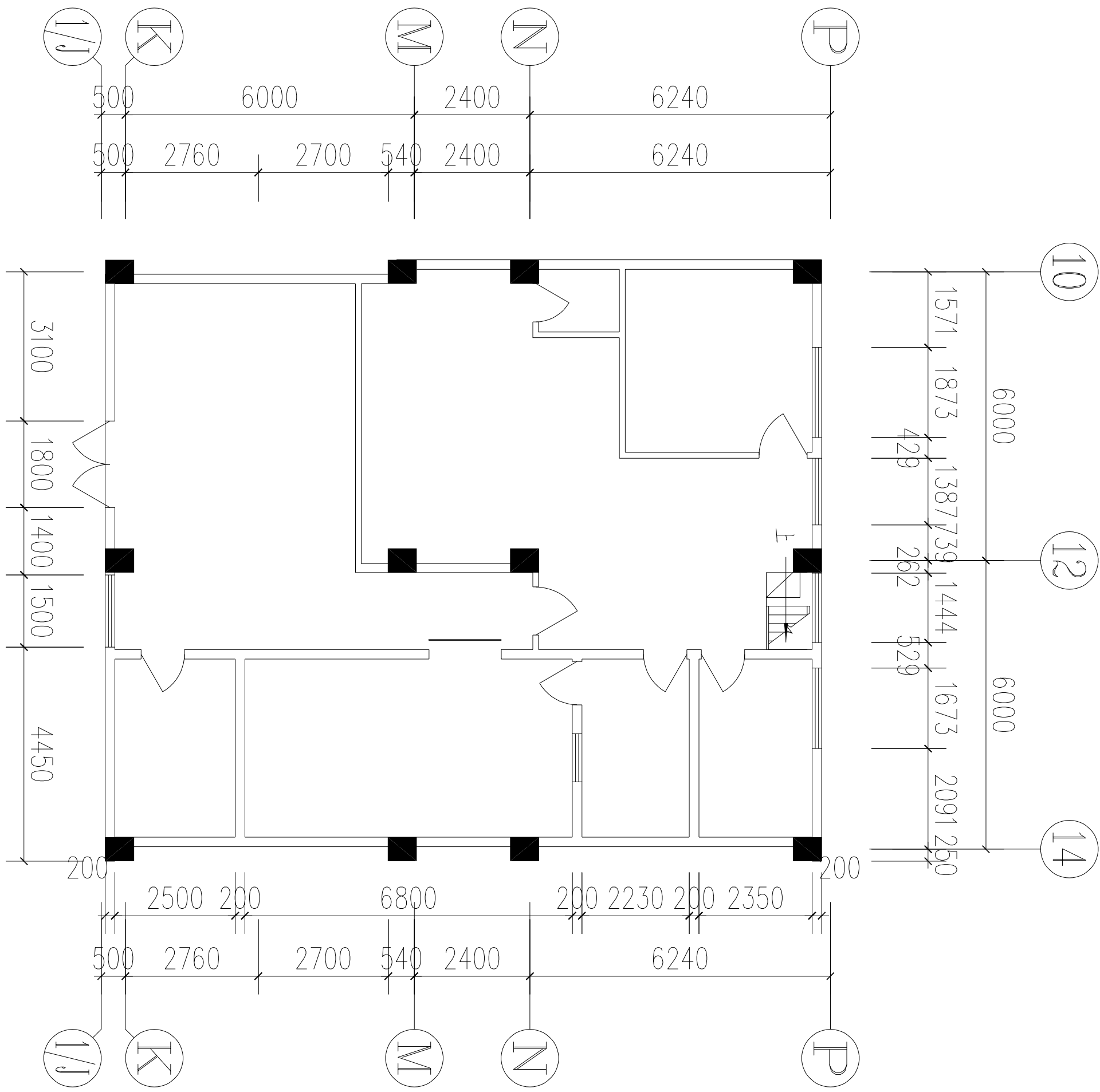
场地现状图
