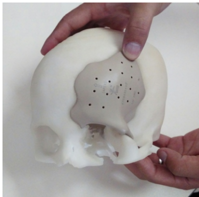
3D打印+聚醚醚酮新材料，无缝结合患者颅骨缺口
